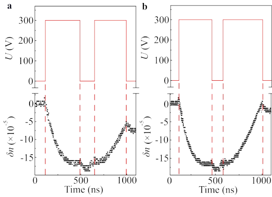
图4 PS-DF-BPLC的 \delta n 随双段电压脉冲的动态响应。第一段电压脉冲时间为400 ns;第二段电压脉冲时间分别为(a)400 ns, (b)550 ns。电场强度 E_0 = 3.8 \times 10^7 V/m, 环境温度 T = 35^\circ\text{C} 。
