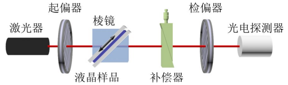
图2 实验装置:用线偏振激光束探测夹在两个直角棱镜之间的液晶盒,该激光束以相对于液晶盒法线的 45^\circ 角度在液晶盒中传播。
