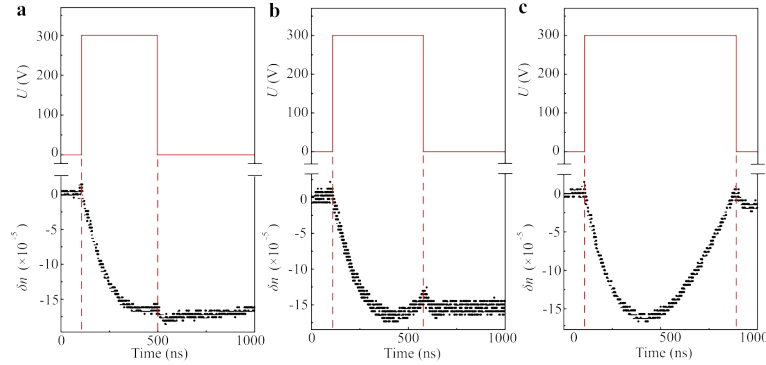
图3 PS-DF-BPLC的 \delta n 随电压脉冲的动态响应。电压脉冲时间分别为(a)470 ns, (b)600 ns, (c)770 ns, 电场强度 E_0 = 3.8 \times 10^7 V/m, 环境温度 T = 35^\circ\text{C} ,
