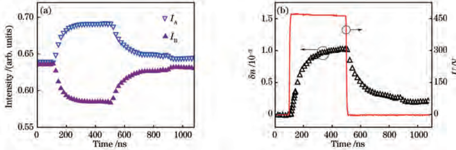
图 2 消双轴入射光路下, 施加的电场引起透射光强与液晶 N2 双折射率的变化 (工作温度为 23 °C, 电压 U_0 = 478 V, 盒厚 d = 4.6 \mu\text{m} )。(a) 纳秒电压脉冲对透射光强的动态作用; (b) 场致双折射率 \delta n 随所加电压 U 的动态变化
